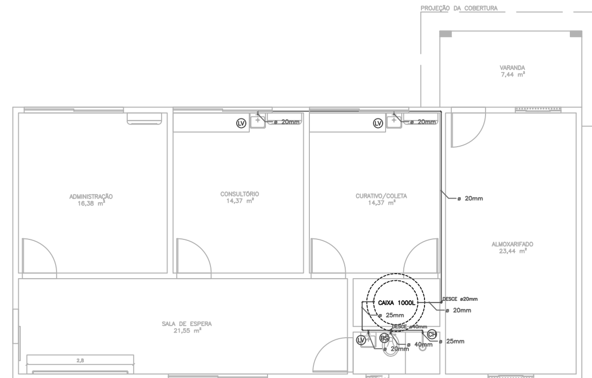
INSTALAÇÃO HIDRAÚLICA ESC.: 1/100
