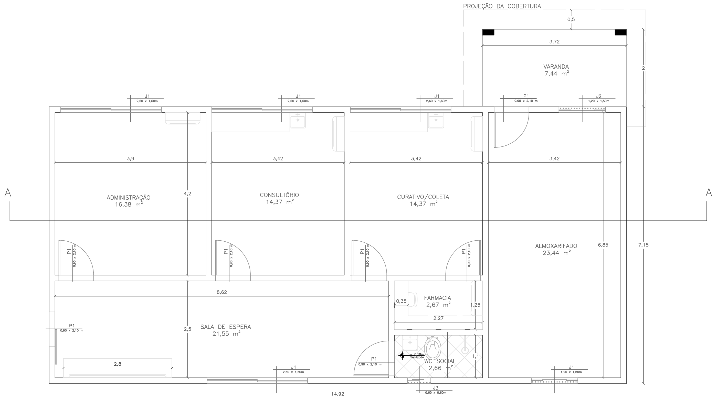
① AMBULÁTORIO-CTV ESC. 1/50
