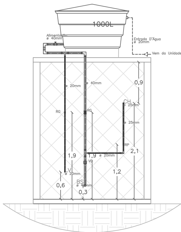
CORTE - INSTALAÇÃO HIDRAÚLICA ESC.: 1/50
