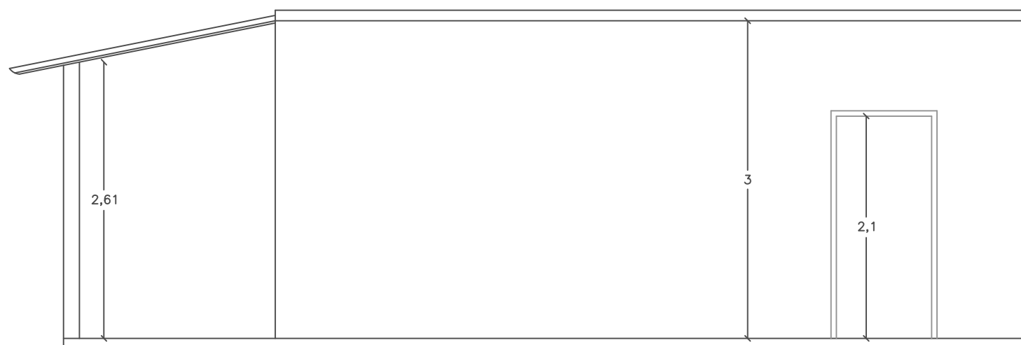
FACHADA ESC.: 1/50
