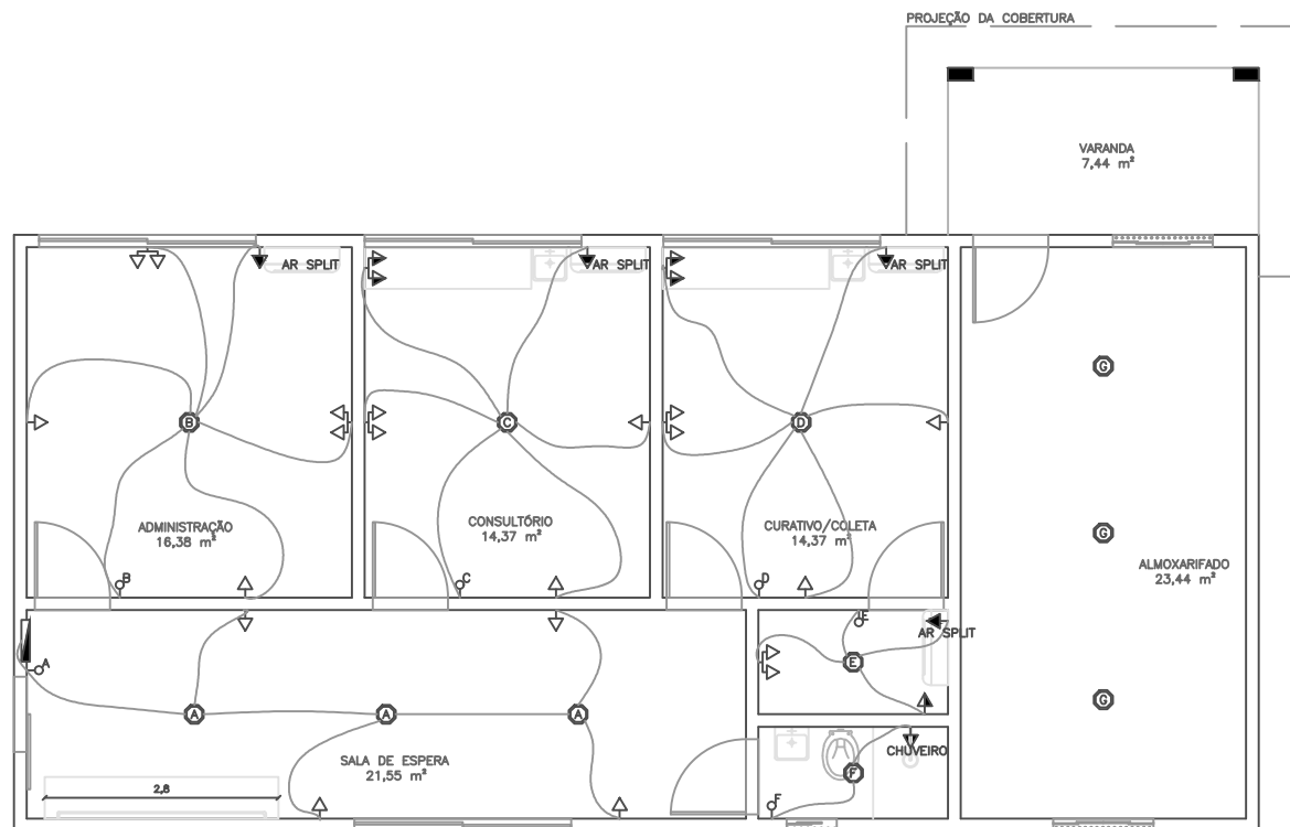
INSTALAÇÃO ELÉTRICA ESC.: 1/100
